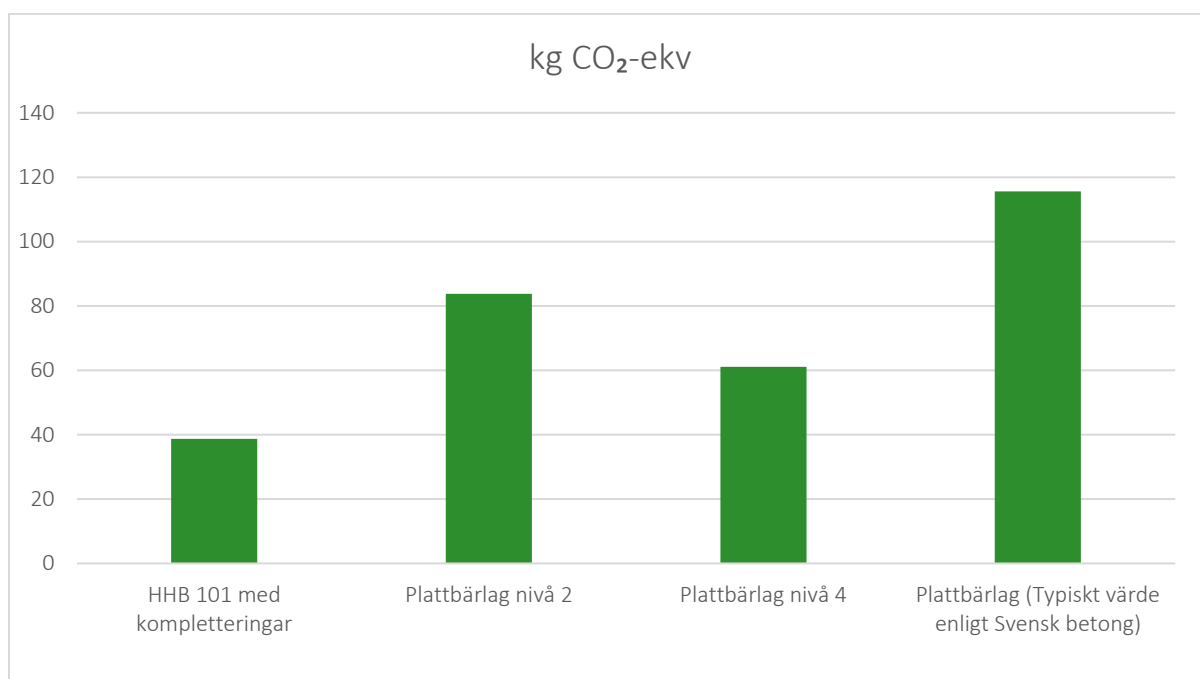
Figur 1: Klimatpåverkan av HHB 101 och olika typer av plattbärlag
