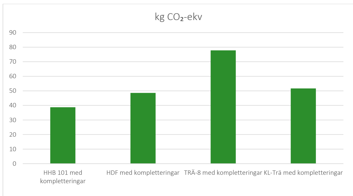
Figur 2: Klimatpåverkan av HHB 101 och olika typer av plattbärlag
